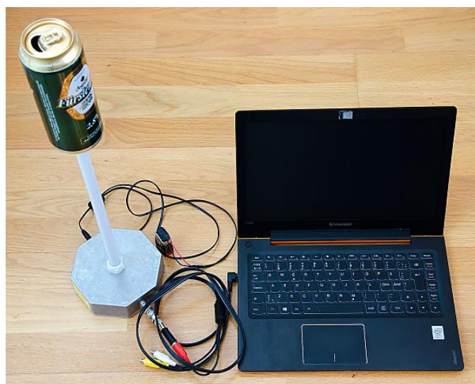
Tonny SA0CLO hade ett intressant föredrag om Grimeton SAQ den 27/10. Han visade också sin berömda "ölburksantenn" med vilken han kunde ta emot SAQ på 17 kHz!
